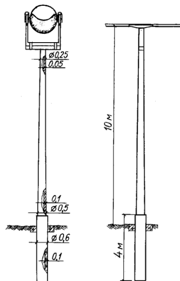
Рис.4. Промежуточная опора малой высоты однопутной СТС
