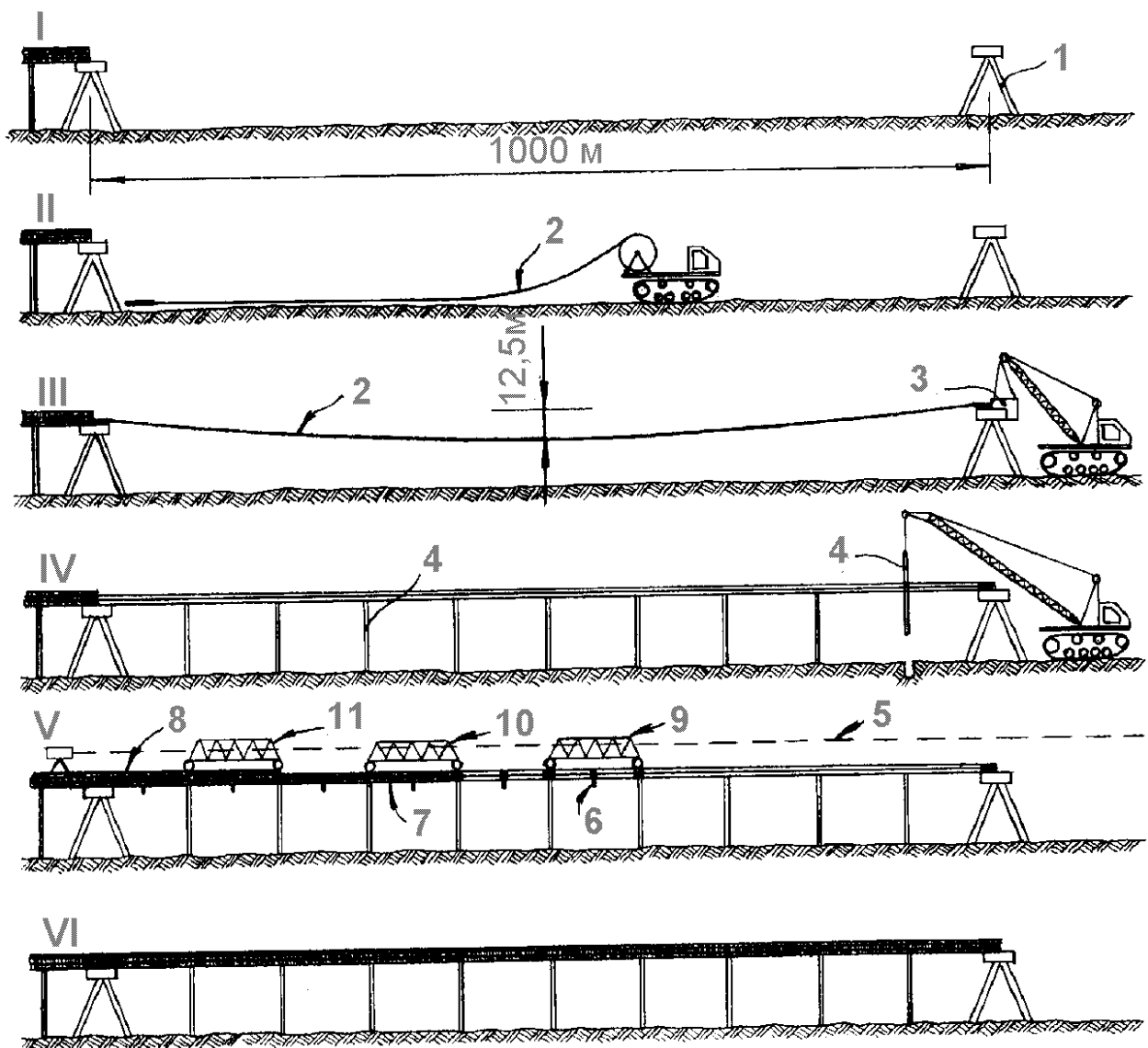
Рис.9. Технология строительства трассы СТС.
