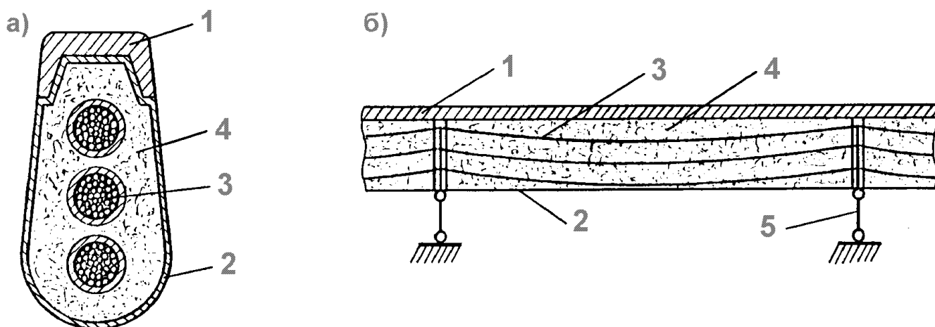
Рис.2. Конструкция рельса-струны:
