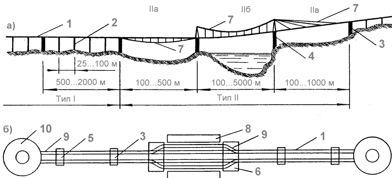
Рис.1. Линейная схема трассы:
