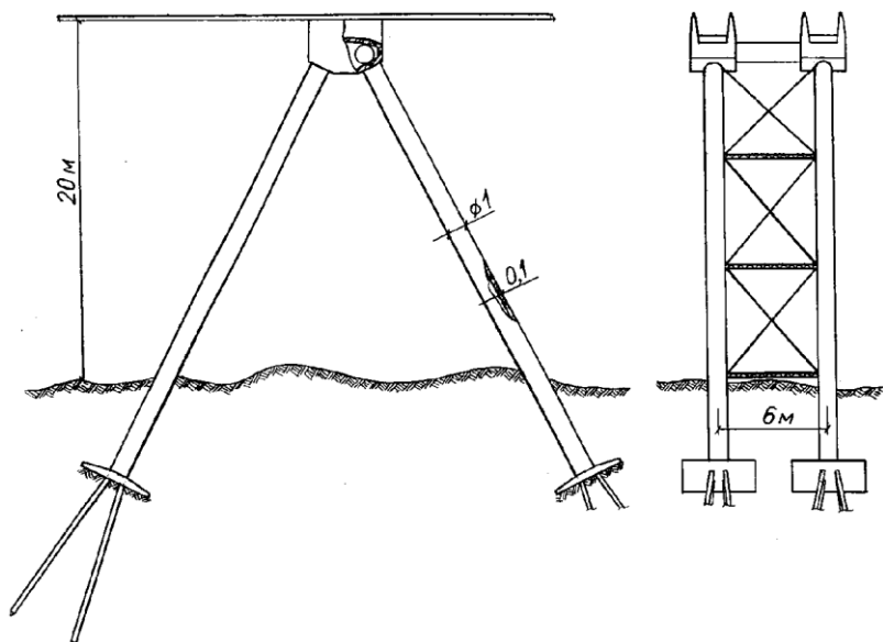
Рис.3. Анкерная опора двухпутной трассы СТС
