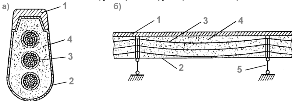
Рис.2. Конструкция рельса-струны:
