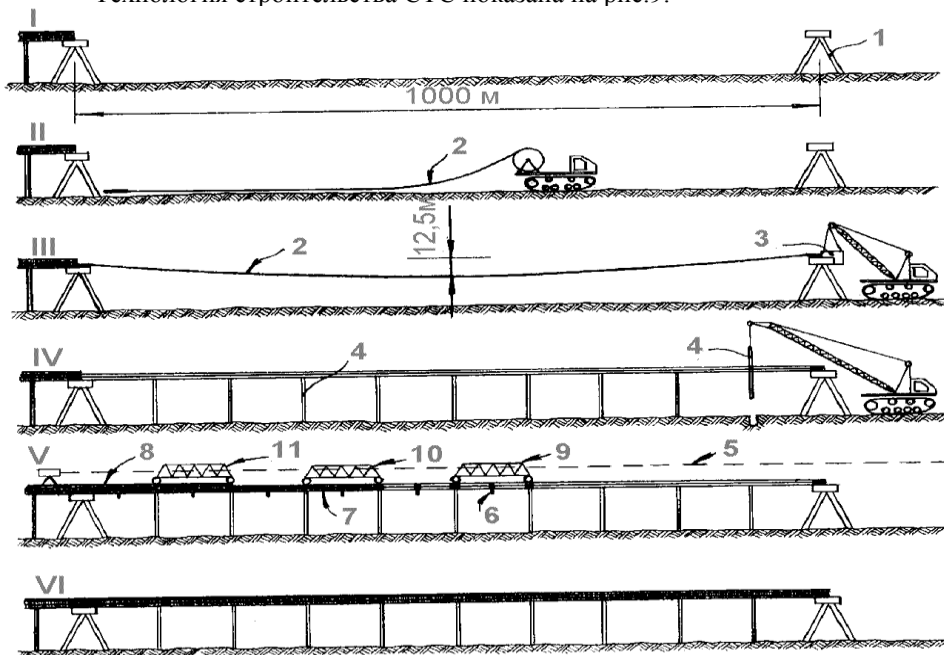
Рис.9. Технология строительства трассы СТС.
