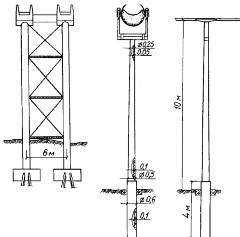
Рис.4. Промежуточная опора малой высоты однопутной СТС
